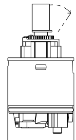
\varnothing 40 \pm 0.2
