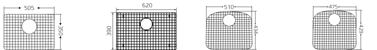
רשת תחתית לכיור ויזן 110 GRID 3 רשת תחתית לכיור קלארון 700 וזירוקס 700 GRID 8 רשת תחתית לכיור דיאמונד GRID 2 רשת תחתית לכיור WAVE GRID 1
