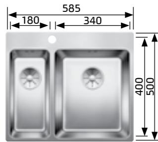
545 - פנימי של שתי הקערות ביחד 340/180-IF/A
