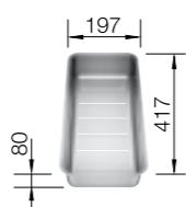
קערית שאריות מנירוסטה 227689
